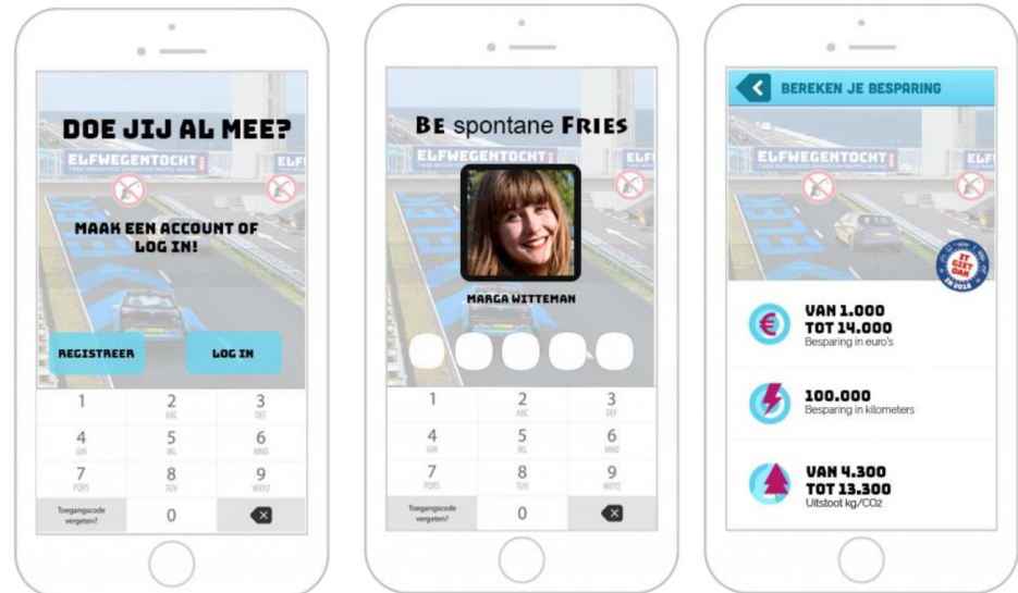
Figuur 8 | App
